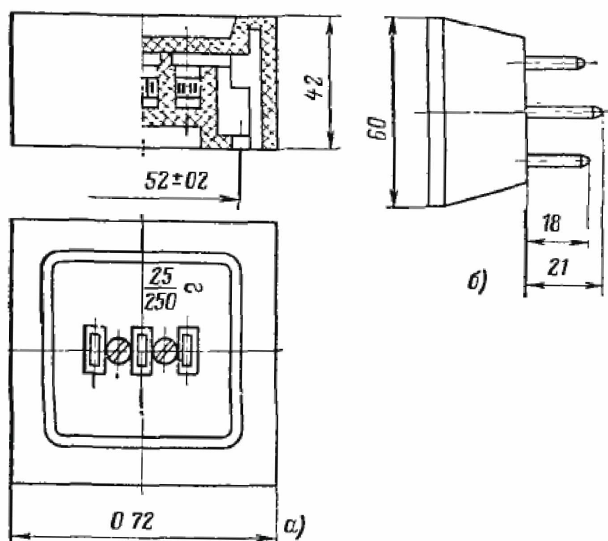
Рис. 18.9. Штепсельное соединение на 25 А с плоскими контактами: а — розетка РШ-20-0-25/250; б — вилка ВШ-20-25/250
