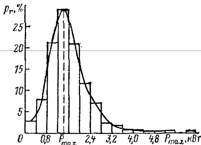
Рис. 3.2. Гистограмма распределения максимумов нагрузки на вводе в квартиру с электроплитой
