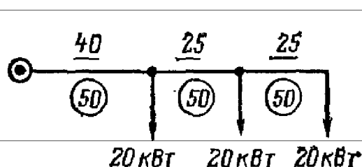
Рис. 11.5. Схема к примеру 11.1. Подчеркнутые цифры — длина, м; в кружках — сечения проводников, \text{мм}^2
