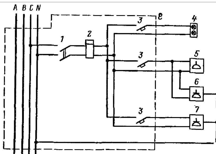
Рис. 7.8. Схема групповой квартирной сети:
