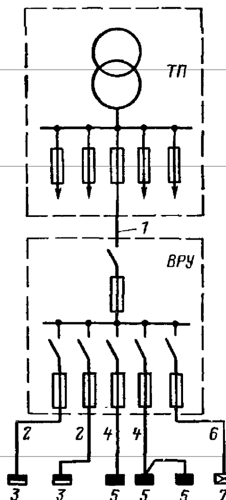
Рис. 8.1. Схема питания общественного здания от однотрансформаторной подстанции
