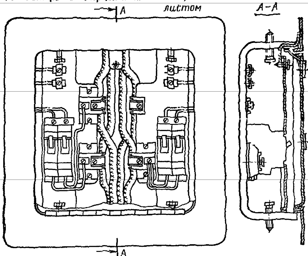
Рис. 17.3. Этажный щиток с аппаратурой защиты
