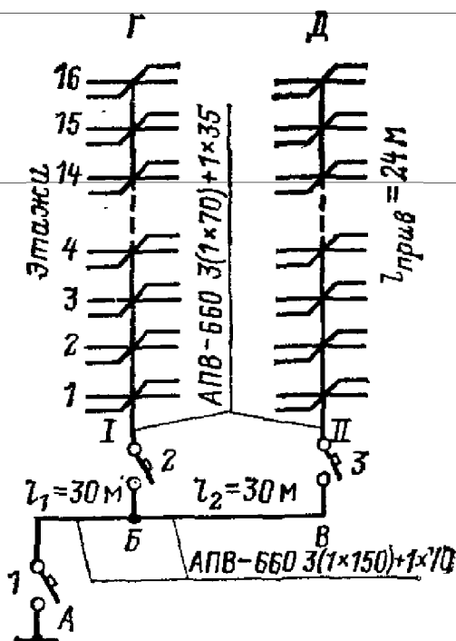
Рис. 11.5. Схема к примеру 11.1. Подчеркнутые цифры — длина, м; в кружках — сечения проводников, \text{мм}^2
