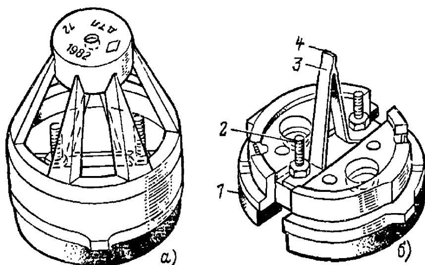
Рис. 22.1. Устройство ДТЛ:
