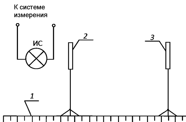
1 – фотометрическая скамья; 2 – шторка; 3 – фотоприемное устройство Рисунок И.1
